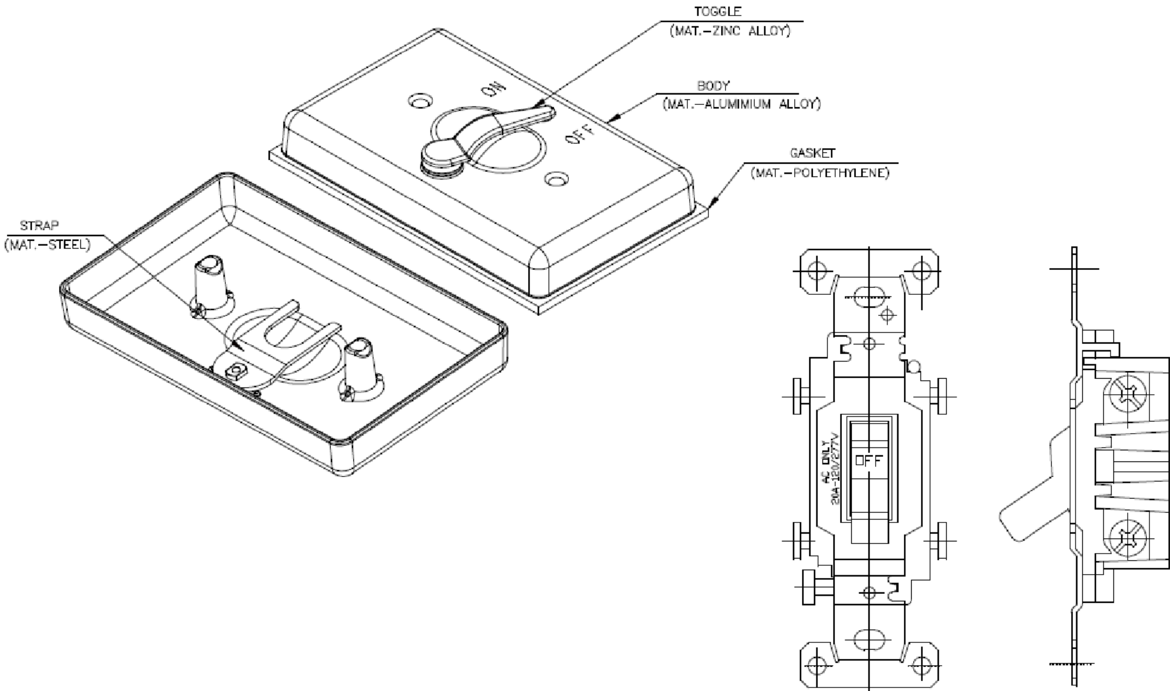
SWITCH TYPE RECEPTACLE DOUBLE POLE
