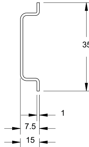
Figure 21. DIN Rail Dimensions
