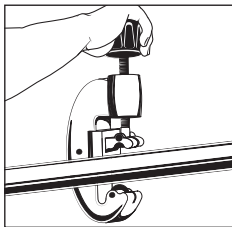
1. Cut tube Corte el tubo
