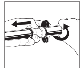
Push the disconnect clip against the release collar and pull the pipe with a twisting action. Empuje el clip de desconexión contra el collar de liberación, y extraiga el tubo con un movimiento giratorio.
