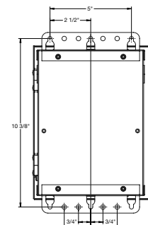
Enceinte intérieure métallique (Kit de montage affleurant IG2200--FMK)
