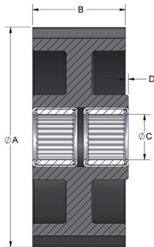
SECTION A-A
