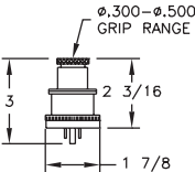
2503B/A-125 2506B/A-125
