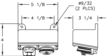
2597B/A-125
